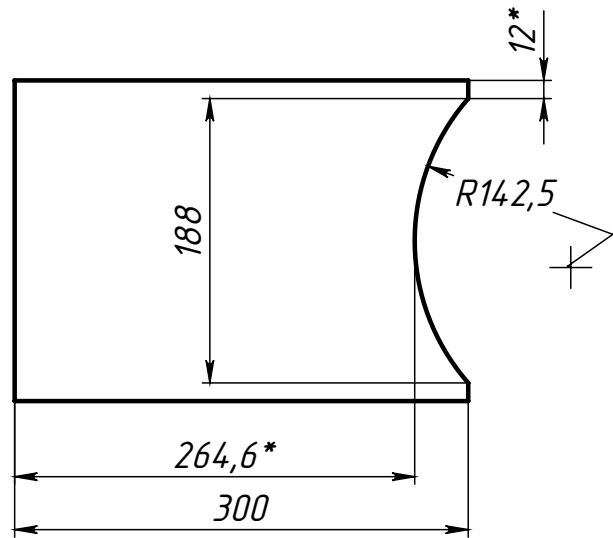
Поз.1 (Основание)
